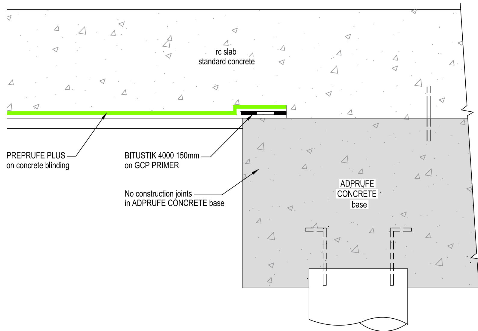
ADPRUFE / PREPRUFE PLUS INTERFACE DETAIL SECTION
